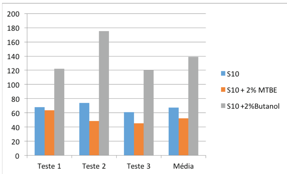
Figura 4 – Variação da turbidez das amostras estudadas
