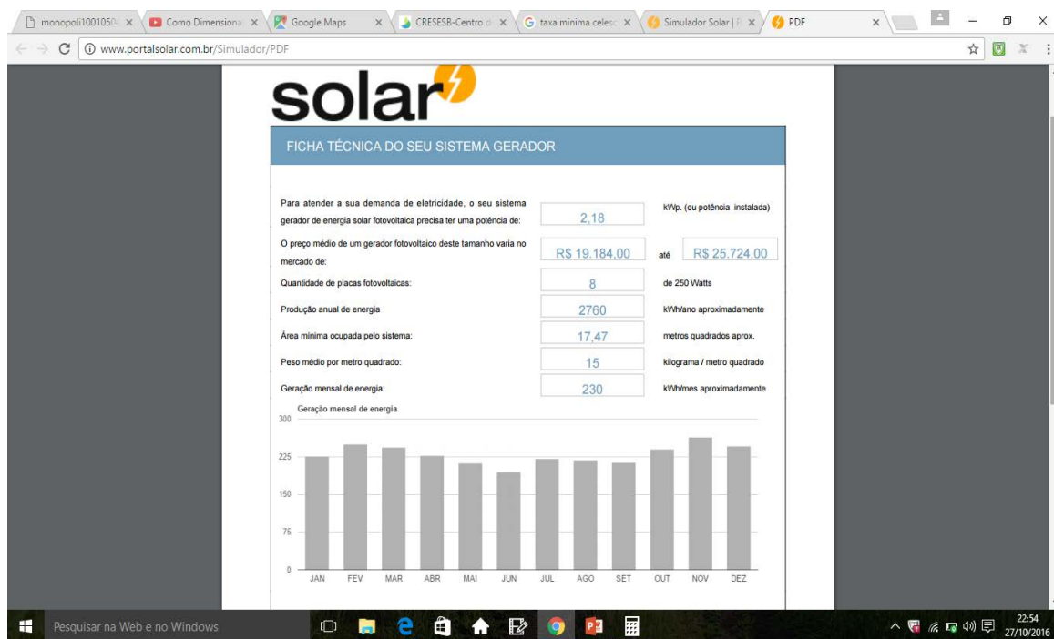
Figura 3 – Dimensionamento e custo de implantação do sistema fotovoltaico numa residência
