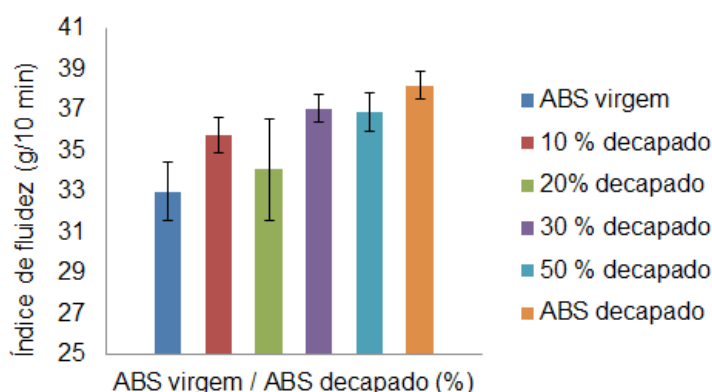
Figura 5 – Índice de fluidez das amostras de ABS virgem, de ABS decapado e das misturas com ABS decapado
