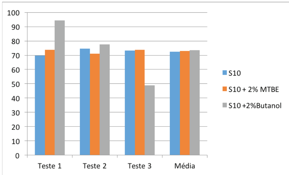
Figura 3 – Variação da concentração de HPA para as condições estudadas
