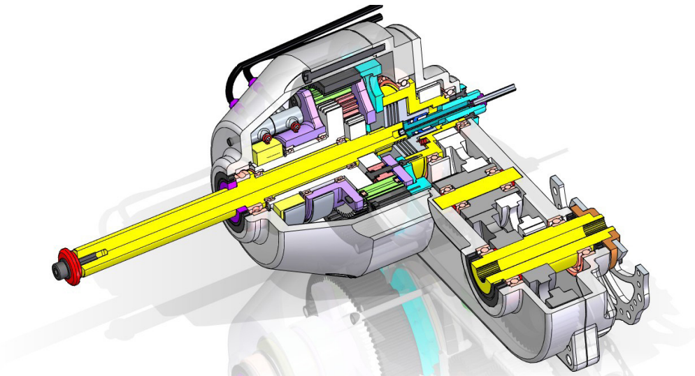
Figura 7 – Conjunto final da transmissão planetária com três marchas
