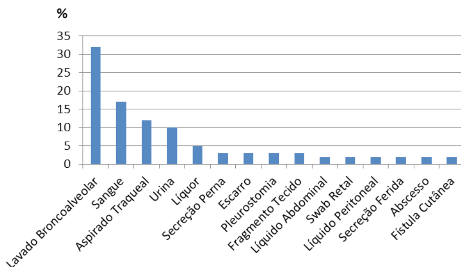
Figura 1 – Tipos de amostras correspondentes aos isolados clínicos do complexo A. calcoaceticus-A. baumannii analisados quanto à ocorrência do gene bla NDM-1
