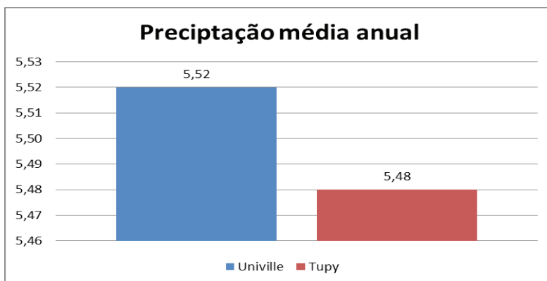
Gráfico 2 – Média mensal de precipitação (mm 3 ) de julho de 2014 a junho de 2015 nas ilhas de calor Univille e Tupy
