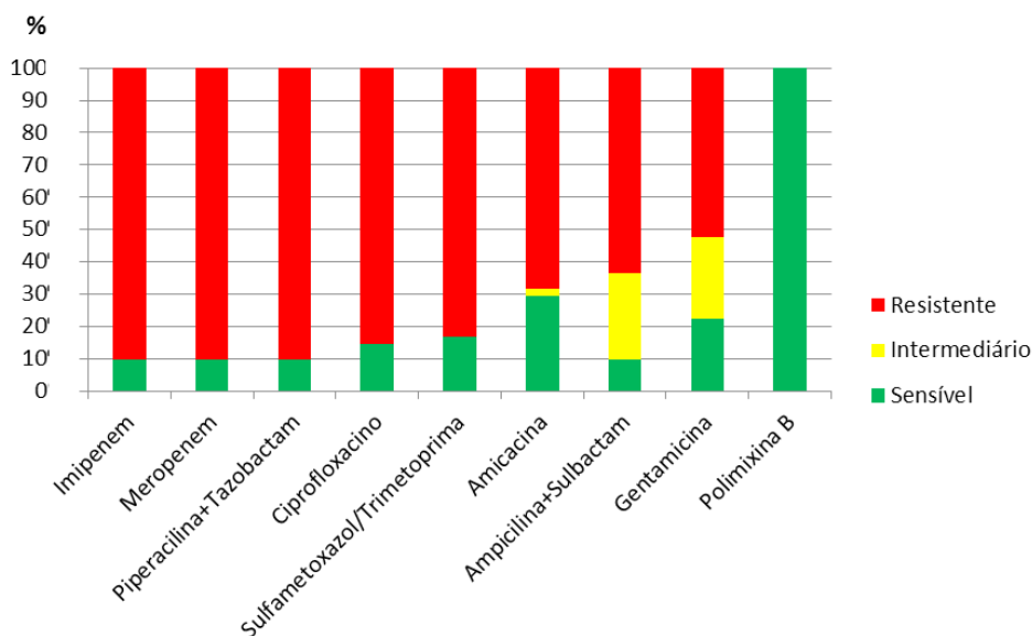
Figura 2 – Perfil de resistência antibiótica in vitro dos isolados clínicos do complexo A. calcoaceticus-A. baumannii analisados quanto à ocorrência do gene bla NDM-1
