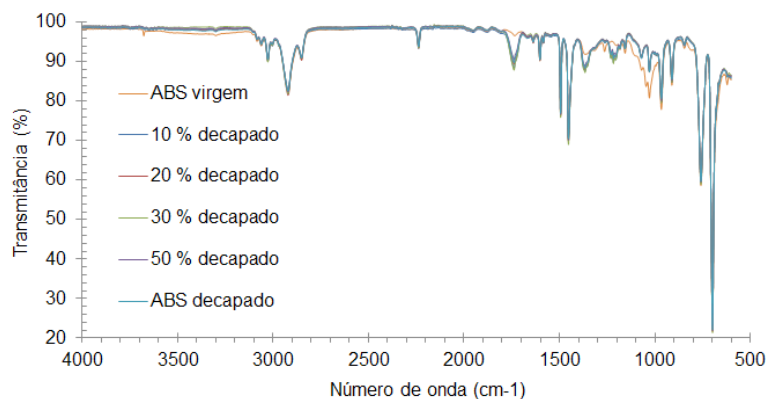
Figura 4 – Espectros FTIR das amostras de ABS virgem, de ABS decapado e das misturas com ABS decapado
