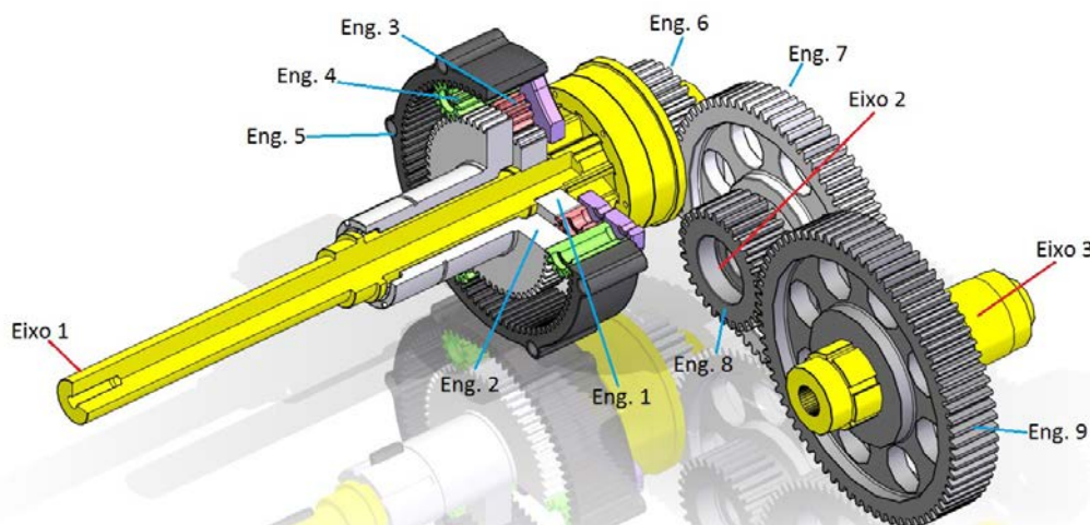
Figura 3 – Leiaute da transmissão e designação de eixos e engrenagens
