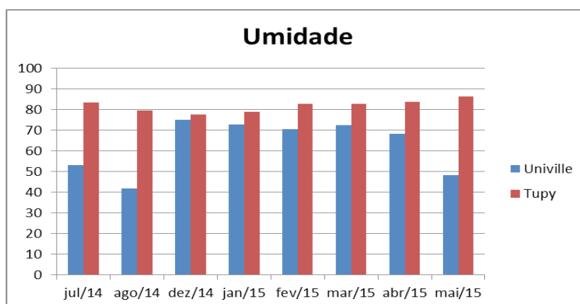
Gráfico 3 – Média mensal de umidade (%) de julho de 2014 a junho de 2015 nas ilhas de calor Univille e Tupy
