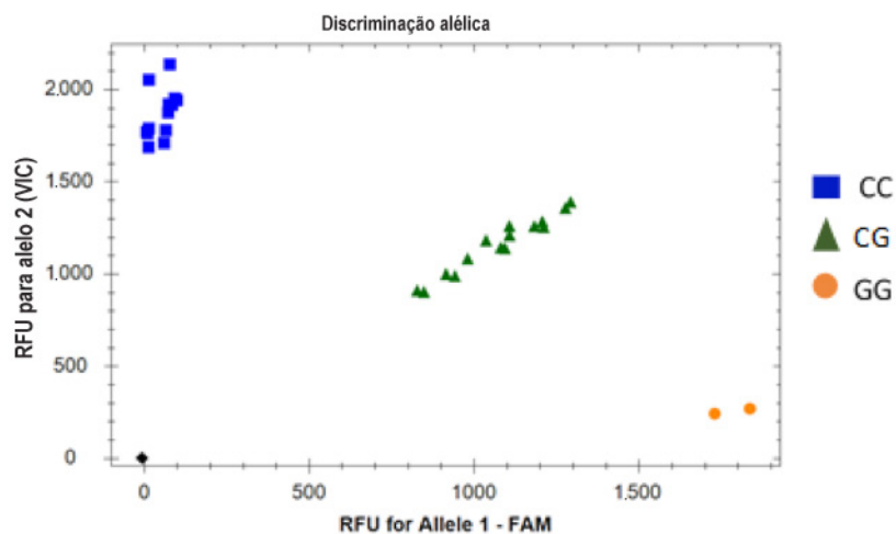
Figura 2 – Representação esquemática da segregação dos resultados de discriminação alélica de um conjunto de resultados de genotipagem do polimorfismo de base única rs738409 do gene PNPLA3
