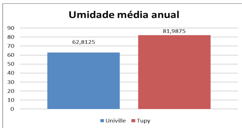
Gráfico 4 – Média anual de umidade (%) de julho de 2014 a junho de 2015 nas ilhas de calor Univille e Tupy
