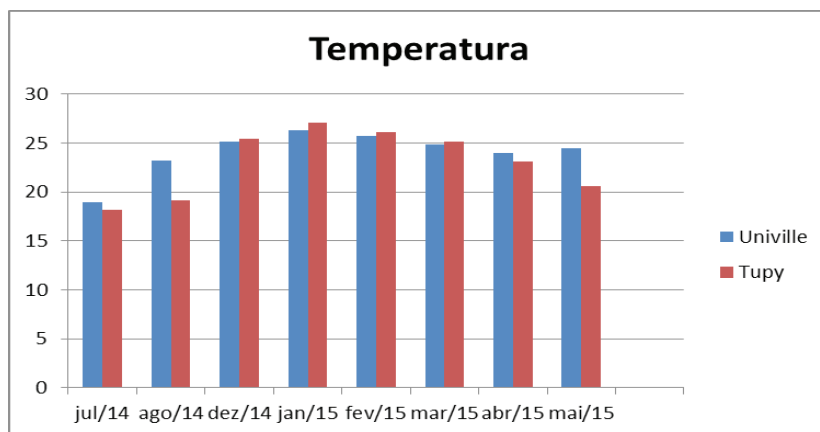
Gráfico 5 – Média mensal (°C) de temperatura de julho de 2014 a maio de 2015 nas ilhas de calor Univille e Tupy
