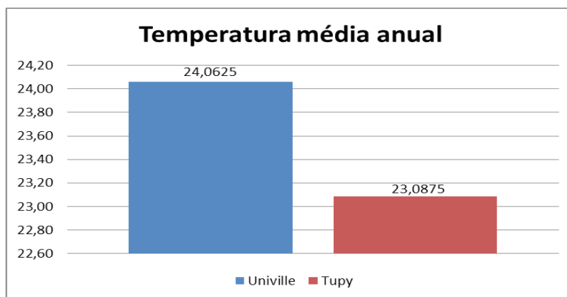
Grafico 6 – Média anual (°C) de temperatura de julho de 2014 a maio de 2015 nas ilhas de calor Univille e Tupy
