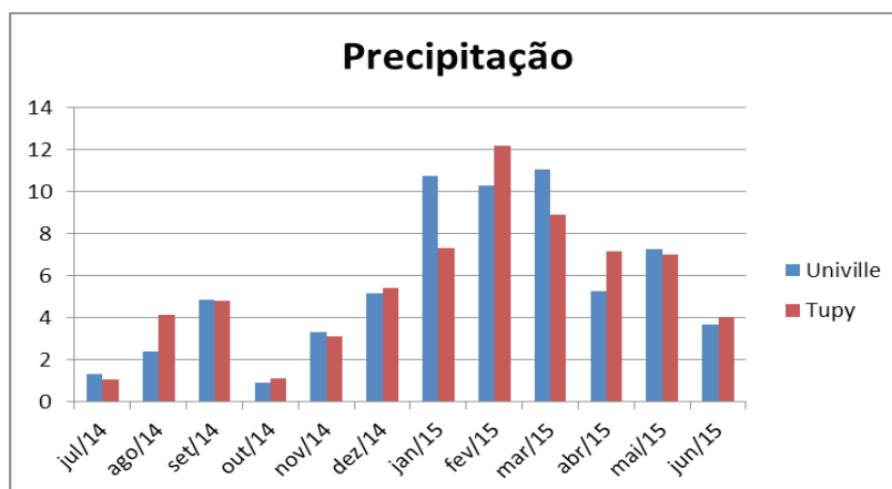
Gráfico 1 – Média mensal de precipitação (mm 3 ) de julho de 2014 a junho de 2015 nas ilhas de calor Univille e Tupy
