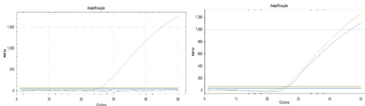
Figura 1 – Perfis de amplificação correspondentes aos genótipos CC (A) e CG (B) do SNP rs738409 do gene PNPLA3
