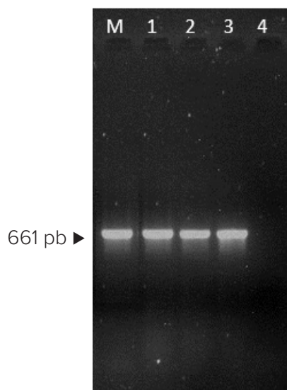
Figura 3 – Padrão eletroforético observado nas amostras analisadas referente à investigação do gene bla NDM-1 por PCR. (M) Amplicon positivo (661 pb); (1) e (2) isolados clínicos bla NDM-1 positivos; (3) cepa controle positivo; (4) controle negativo da PCR
