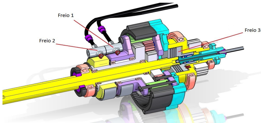
Figura 5 – Sistema proposto para troca de marchas
