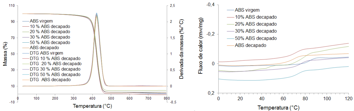
Figura 3 – Curvas de TG/DTG (A) e DSC (B) das amostras de ABS virgem, ABS decapado e das misturas de ABS decapado em diferentes proporções
